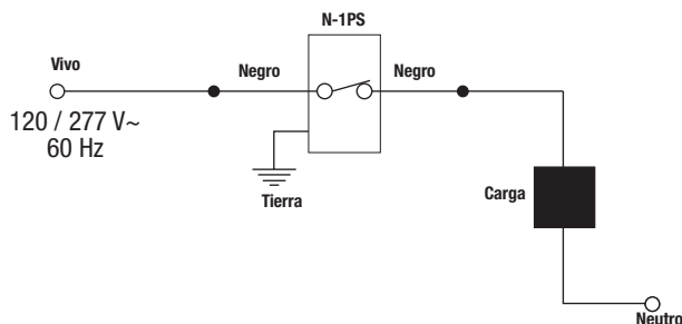
Figura A. Diagrama de cableado. Unipolar.
