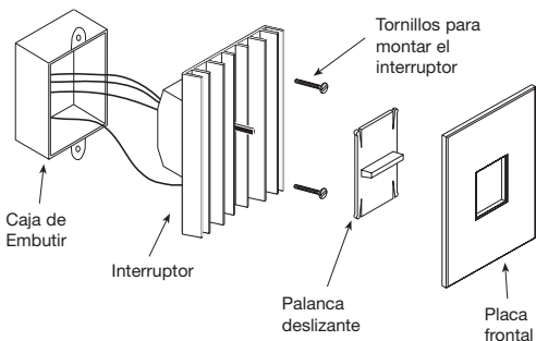
Figura D. Diagrama de montaje
