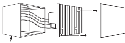
2口用深型ボックス使用の事 (深さ45~55mm程度)
