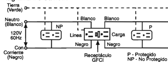
Diagrama De Cableado N° 5
