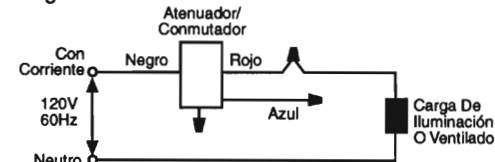
Diagrama De Cableado N° 13
