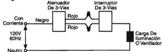
Diagrama De Cableado N° 2
