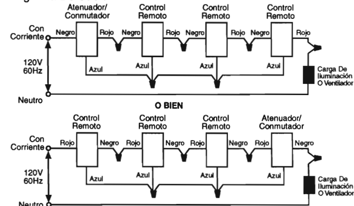
Diagrama De Cableado N° 14
