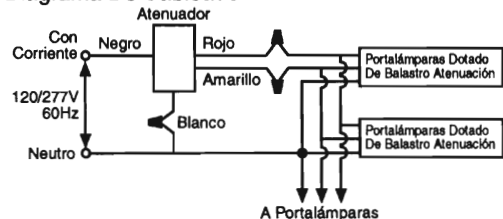
Diagrama De Cableado N° 8
