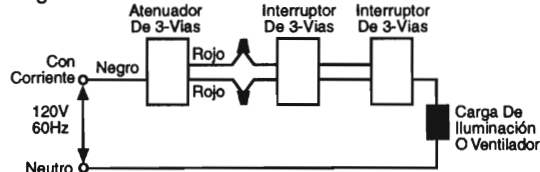
Diagrama De Cableado N° 3
