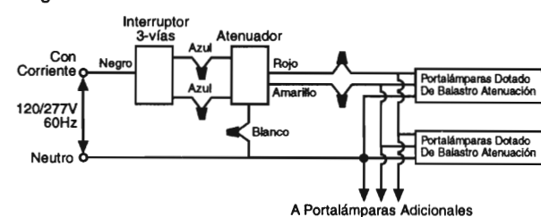
Diagrama De Cableado N° 14
