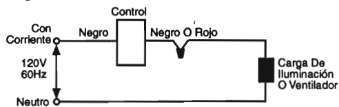
Diagrama De Cableado N° 2
