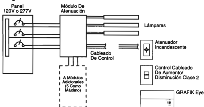
Diagrama De Cableado N° 11
