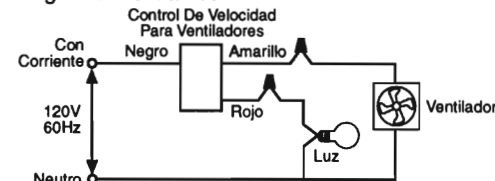
Diagrama De Cableado N° 12
