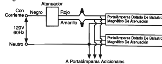
Diagrama De Cableado N° 10
