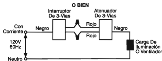
Diagrama De Cableado N° 3
