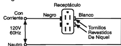
Diagrama De Cableado N° 4
