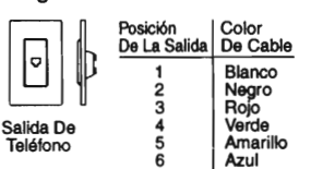
Diagrama De Cableado N° 8
